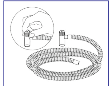
NEOPUFF T PARÇA RESÜSİTASYON DEVRESİ
